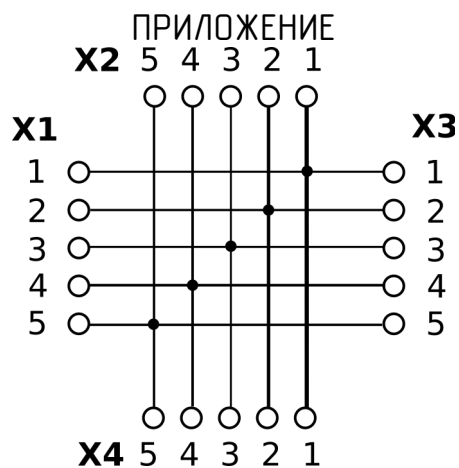
Рис. 1. Схема принципиальная ПР-4.
